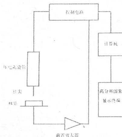
图1 扫描隧道显微镜仪器框图
